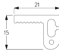
SG 11421 ジップレール
