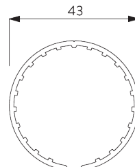
SG 10532 チューブ ø 43 mm
