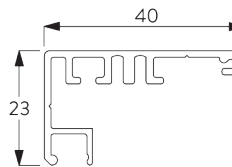
SG 11418 サイドガイドケース
