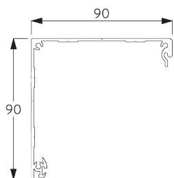
SG 10996 ボックススペース 90 mm
