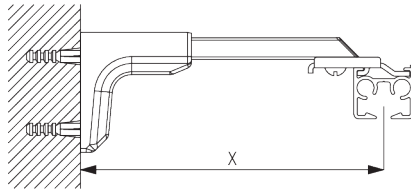
ユニバーサルスマートフィックスセット SG 11156 & ブラケット SG 3832: 必要部品 ボルトネジ SG 10407 (M4x10)
