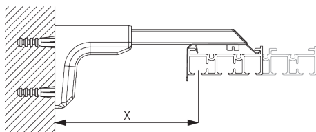
ユニバーサルスマートフィックスセット SG 11156: ブラケット SG 10136 & レール 2 ch ブラケット SG 10137 & レール 3 - 5 ch 必要部品 ボルトネジ SG 10492 (M4x8)
