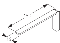
SG 11204 スマートフィックスセット 150 mm
