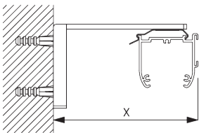
スマートフィックス SG 11200 - SG 11204 & ブラケット SG 2616: 必要部品 ボルトネジ SG 10395 (M4x6)
