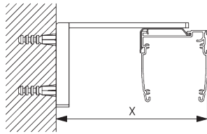
スマートフィックス SG 11200 - SG 11204 & ブラケット SG 2521: 必要部品 ボルトネジ SG 10395 (M4x6)
