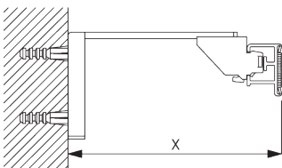
スマートフィックス SG 11200 - SG 11204 & ブラケット SG 3603: 必要部品 ボルトネジ SG 10492 (M4x8)
