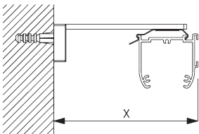
スクエアスマートフィックス SG 11210 - SG 11214 &ブラケット SG 2616: 必要部品 ボルトネジ SG 10395 (M4x6)
