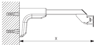
ユニバーサルスマートフィックス SG 11156 & ブラケット SG 3603: 必要部品 ボルトネジ SG 10277 (M4x12)
