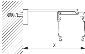
スクエアスマートフィックス SG 11210 - SG 11214 & ブラケット SG 2521: 必要部品 ボルトネジ SG 10395 (M4x6)
