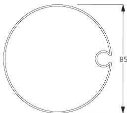
SG 8601 チューブ φ 85 mm
